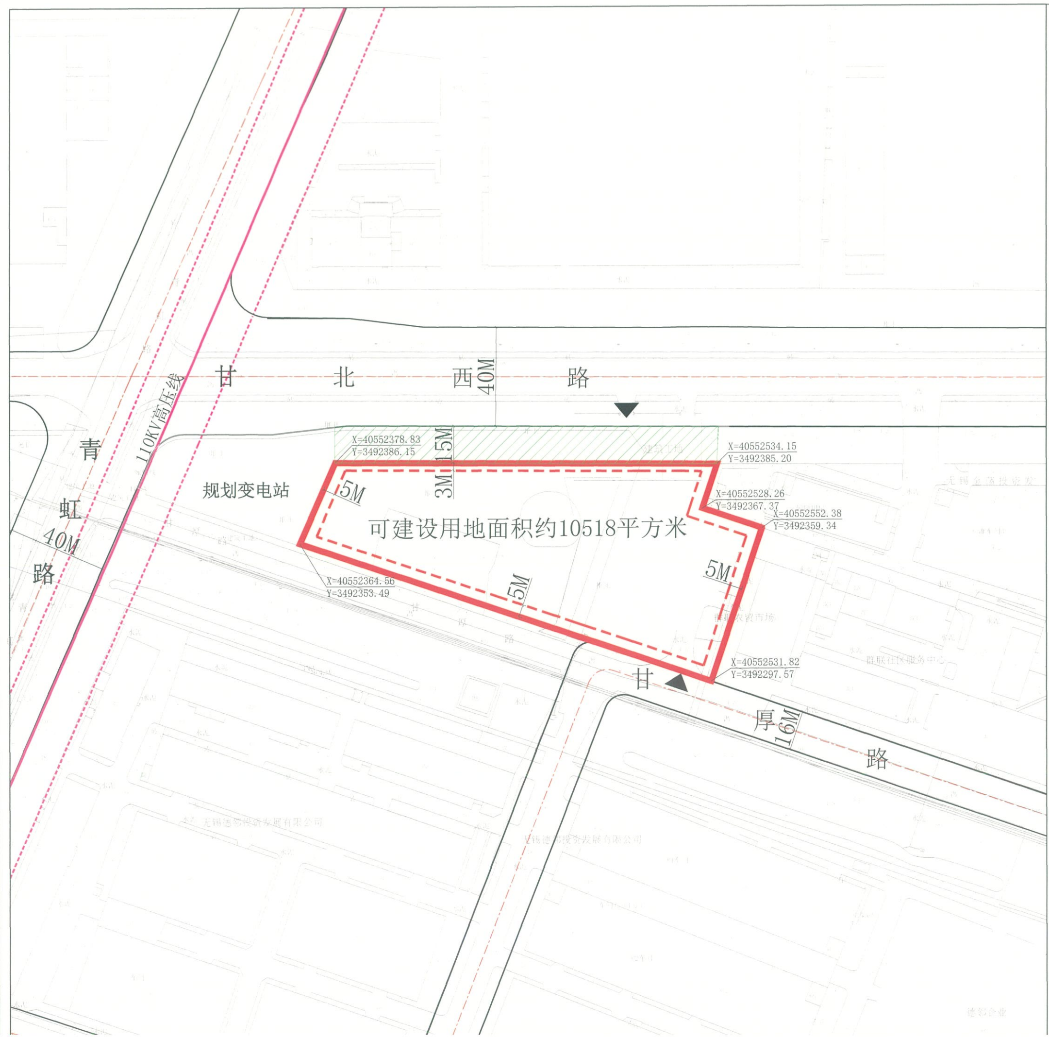
地块区位图
